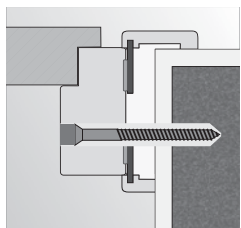
Beépítés purhabbal és dübellel kőműves falba
